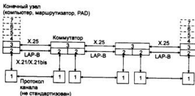
Рис. 2. Стек протоколов сети X.25
