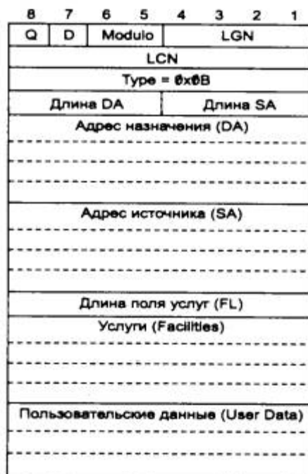
Рис. 3. Формат пакета Call Request
