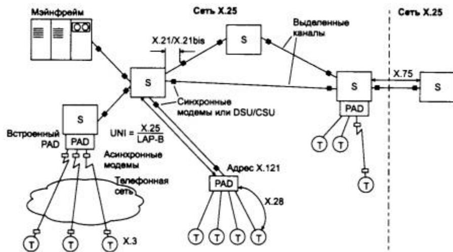
Рис. 1. Структура сети X.25
